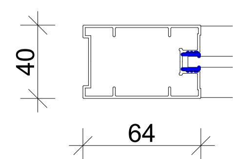
Det.3 / Alt dörr-ram
